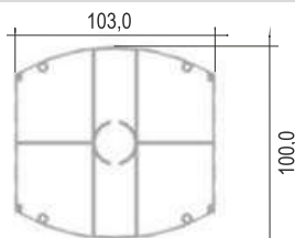
Corte do Perfil do Totem Plus Standard
